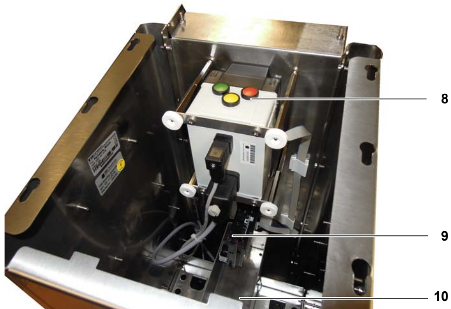
Abb. 2-4 Innenansicht der Parksäule Einfahrt (Frontseite)
