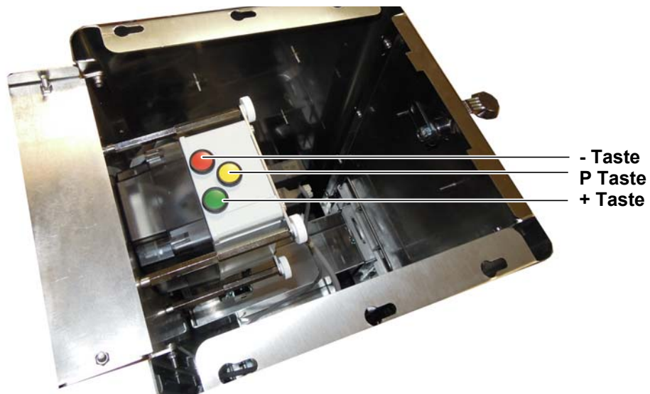
Abb. 7-3 Tastenbelegung Programmierschalter
