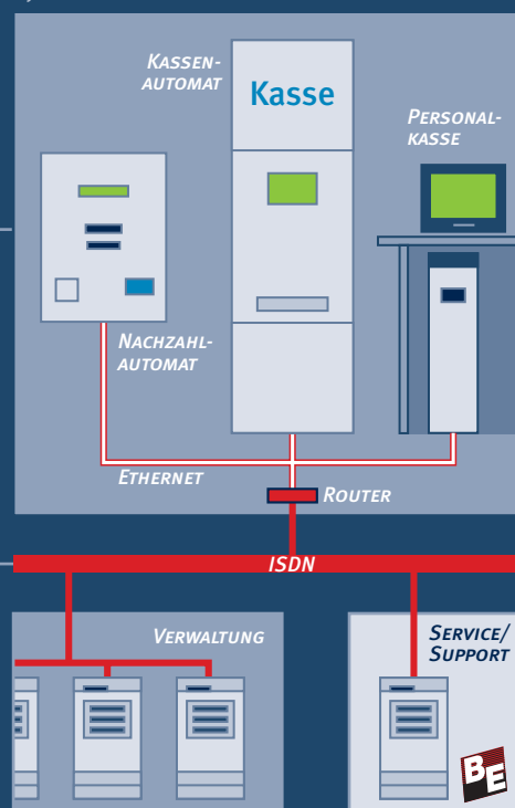
System-Netzwerk
